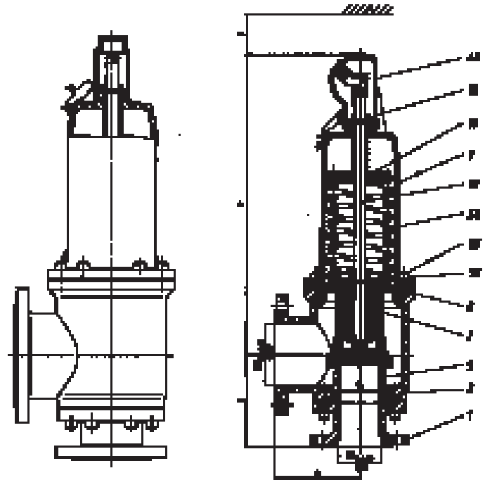
Type 447 mit gasdichter Kappe H 2 with gastight cap H 2
