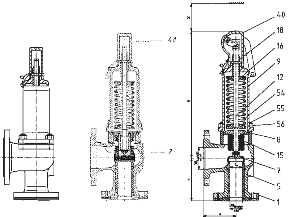
Type 546 mit gasdichter Kappe H 2 with gastight cap H 2
